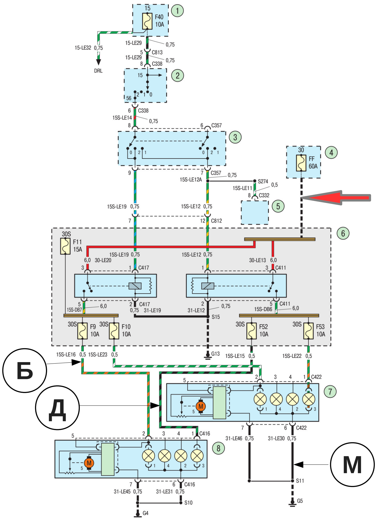
Схема 20а. Блок-фары: 1, 6 – монтажный блок предохранителей и реле за вещевым ящиком; 2 – блок переключателя наружного освещения; 3 – левый подрулевой переключатель; 4 – монтажный блок предохранителей в моторном отсеке; 5 – комбинация приборов; 7 – правая блок-фара; 8 – левая блок-фара
