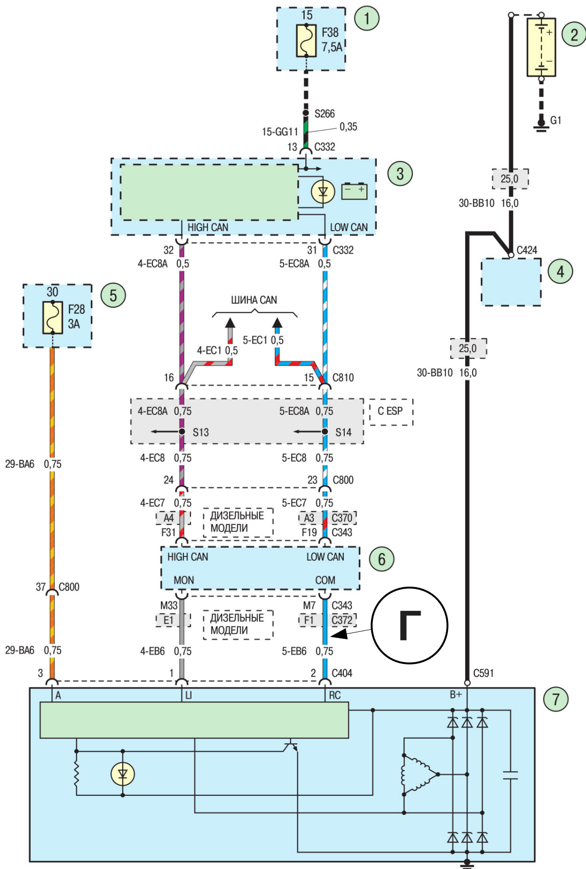
Схема 3а. Система зарядки: 1, 5 – монтажный блок предохранителей и реле за вещевым ящиком; 2 – аккумуляторная батарея; 3 – комбинация приборов; 4 – стартер; 6 – электронный блок управления двигателем; 7 – генератор
